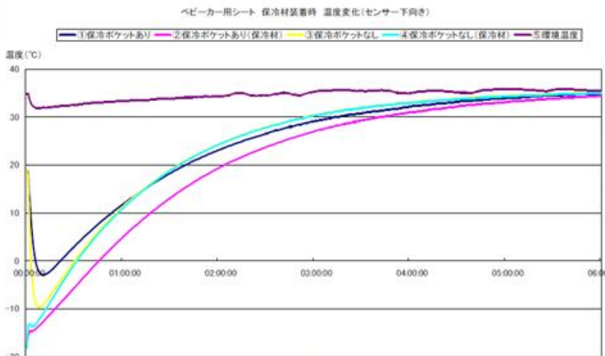
アルミポケット装着時と、そうでない時の保冷剤の温度をあらわしたグラフ
